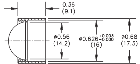
A08086 Input Lens Diffuser
